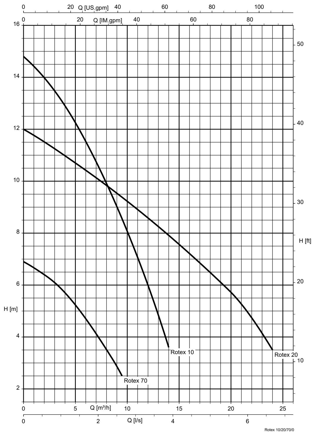
Abb. 1: Freier Kugeldurchgang: Rotex 10 = 10 mm; Rotex 20 = 13 mm; Rotex 70 = 18 mm
