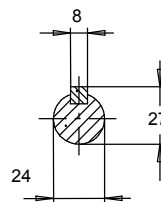
Wellenende Paßfeder nach DIN 6885, B11
