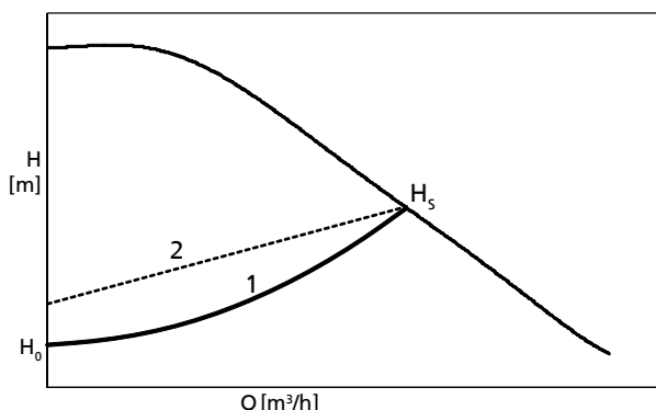
Abb. 1: Funktion Eco-Mode
