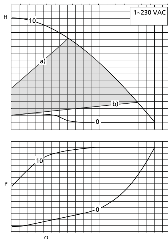
Abb. 3: Auslegungsbeispiel
