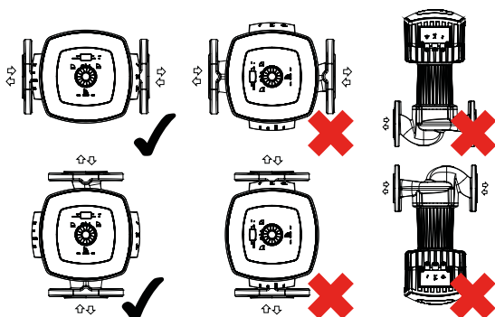
Abb. 6: Zulässige Einbaulagen
