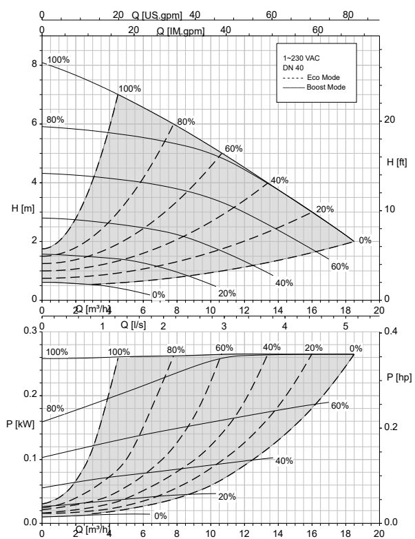
Calio 40-80 Stellerbetrieb, Eco-Mode
