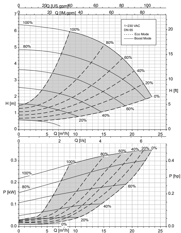
Calio 65-120 Stellerbetrieb, Eco-Mode
